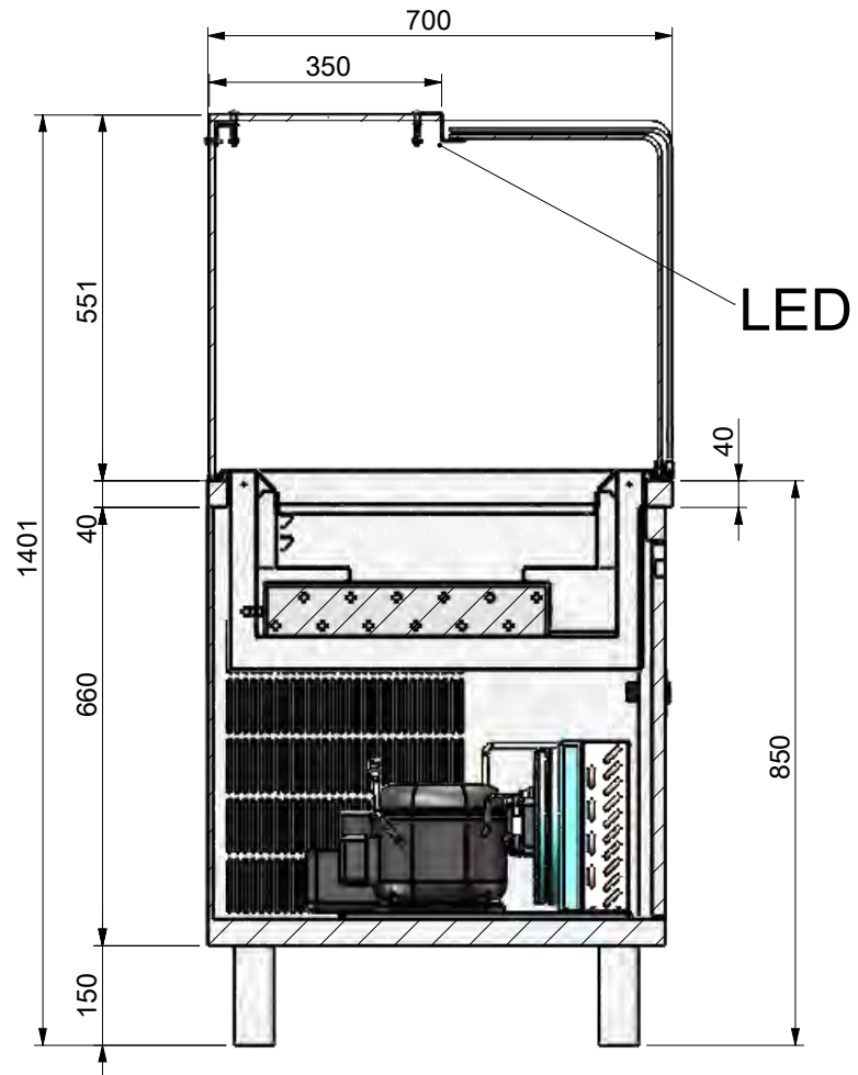
SEZIONE D-D
