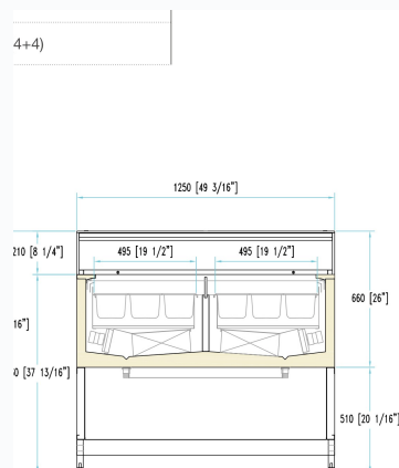
VUE DE FACE (cotes constructeur)
