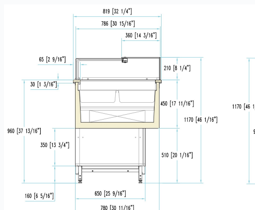
VUE DE CÔTÉ (cotes constructeur)
