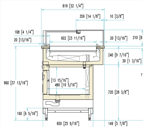
VUE DE CÔTÉ (cotes constructeur)
